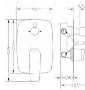
Ref.: 62118 08 45 66 Monomando empotrado con inversor cerámico 3 vías Built-in single handle mixer with 3 way ceramic diverter
