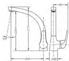
Ref.: 61203 06 45 66 Monomando de fregadera caño conformado Single-lever sink mixer tube spout
