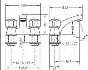
Ref.: 68122 11 45 66 Mezclador lavabo centerset 4" Wash-basin mixer 4" centerset
