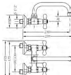
Ref.: 68560 09 45 66 Grupo mural fregadera 15cm caño tubo bajo 24cm Wall sink mixer 15cm low tube spout 24cm
