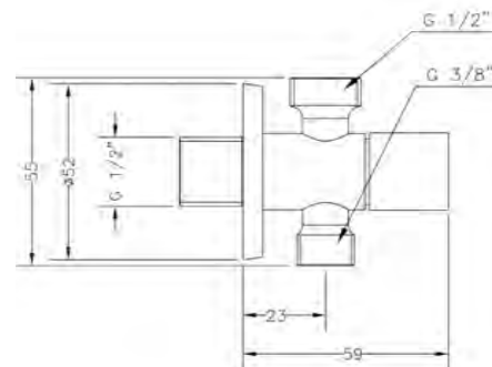
Ref.: 3107 03 Válvula de escuadra doble 1/2\"/>
