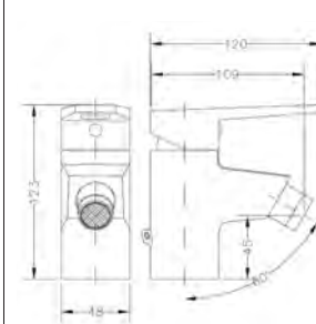
Ref.: 64140 14 45 66 Monomando de bidé Single lever bidet mixer
