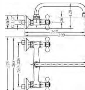
Ref.: 68565 09 45 66 Grupo mural fregadera 20 cm caño tubo alto 24cm Wall sink mixer 20cm high tube spout 24cm
