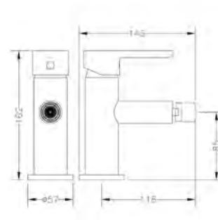
Ref.: 65140 19 45 66 Monomando de bidé Single lever bidet mixer
