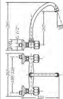
Ref.: 68103 11 45 66 Grupo mural fregadera 20 cm caño tubo alto vertical Wall sink mixer 20cm swan neck spout
