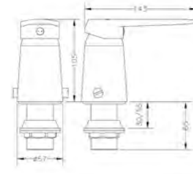
Ref.: 62142 31 45 66 Monomando de bidé con transmisión Single lever bidet mixer with diverter
