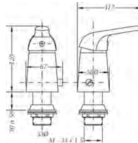
Ref.: 61142 06 45 66 Monomando de bidé con transmisión Single lever bidet mixer with diverter
