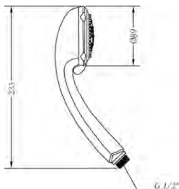
Ref.: DXE5 45 Mango de ducha E5 jets (caja) E5 jets handshower (box)
