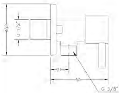
Ref.: 3104 04 Válvula de escuadra redonda 3/8\"/>
