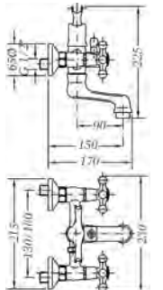
Ref.: 68526 09 43 66 Mezclador de baño bronce con kit Bath mixer bronze with kit
