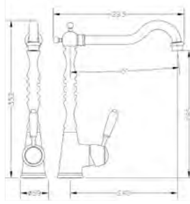
Ref.: 68201 39 45 66 Monomando de fregadera cromo cartucho 40 Sink mixer chromed 40 cartridge
