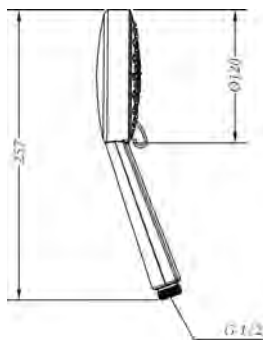
Ref.: DXT5 45 Mango de ducha T5 jets (caja) T5 jets handshower (box)
