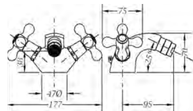
Ref.: 68515 09 45 66 Monobloc de bidé Bidet mixer
