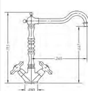
Ref.: 68595 09 45 66 Monobloc de fregadera cromo Sink mixer chromed
