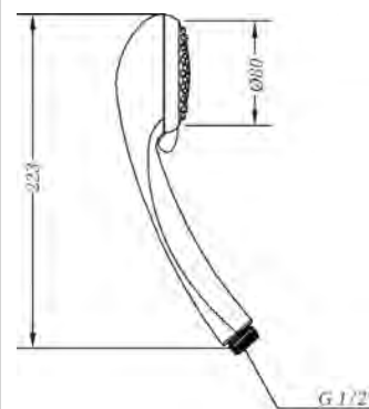
Ref.: DXE2 45 Mango de ducha E2 jets (caja) E2 jets handshower (box)
