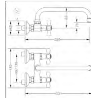
Ref.: 68196 09 45 66 Grupo mural fregadera 11 cm caño tubo alto 24cm Wall sink mixer 11cm high tube spout 24cm
