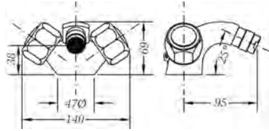
Ref.: 68140 11 45 66 Monobloc de bidé Bidet mixer
