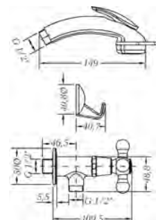
Ref.: 68001 09 45 66 Grifo de bide con teleducha Bidet tap with shower
